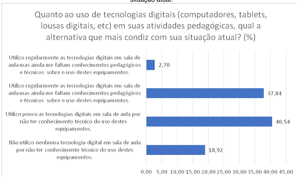
Gráfico 13 – Questão 2.3: quanto ao uso de tecnologias digitais (computadores, tablets, lousas digitais, etc) em suas atividades pedagógicas, assinale a alternativa que mais condiz com sua situação atual:
